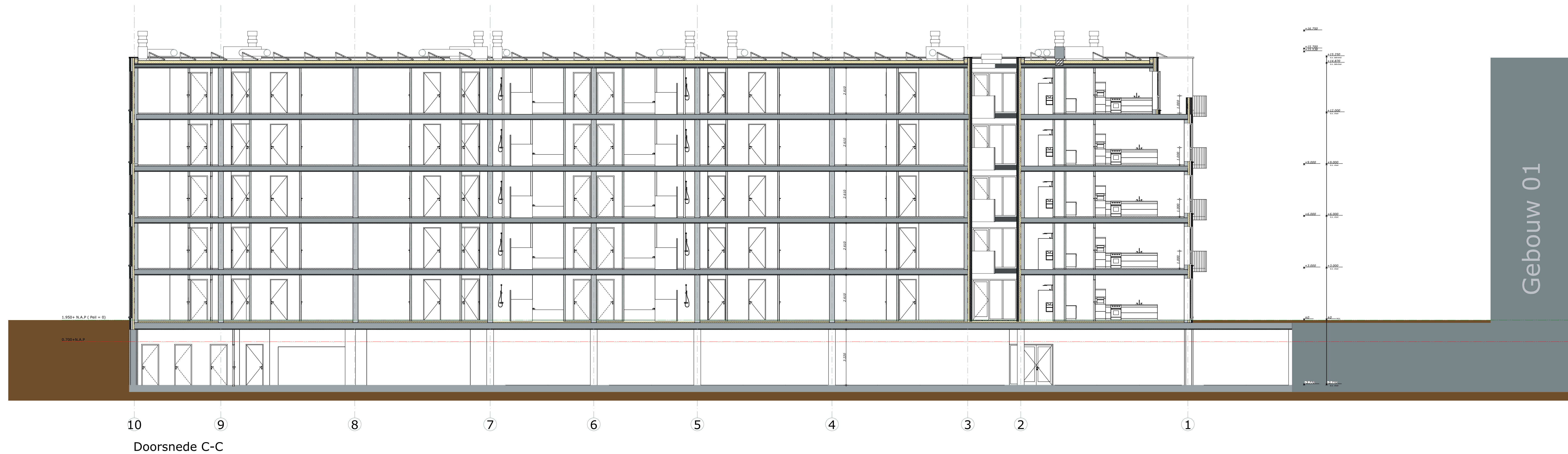
Doorsnede C-C
